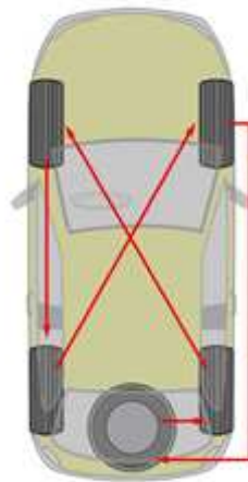
Rotacion de 5 neumaticos – Todos de la misma medida y construccion diagonal
