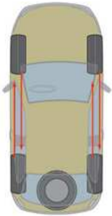
Rotación de 4 Neumáticos – Todos de la misma medida y construcción radial
